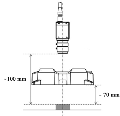
图 5 光源与相机安装示意图
