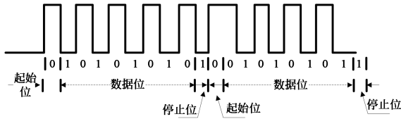
图 8 RS232 数据传输时序图
